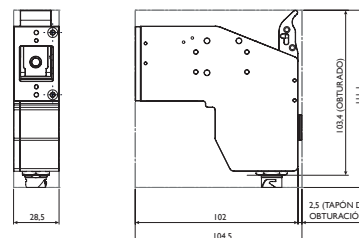
Cabezal de impresión compacto de la Serie Gx
