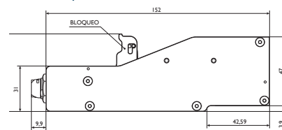
Cabezal de impresión compacto de la Serie Gx
